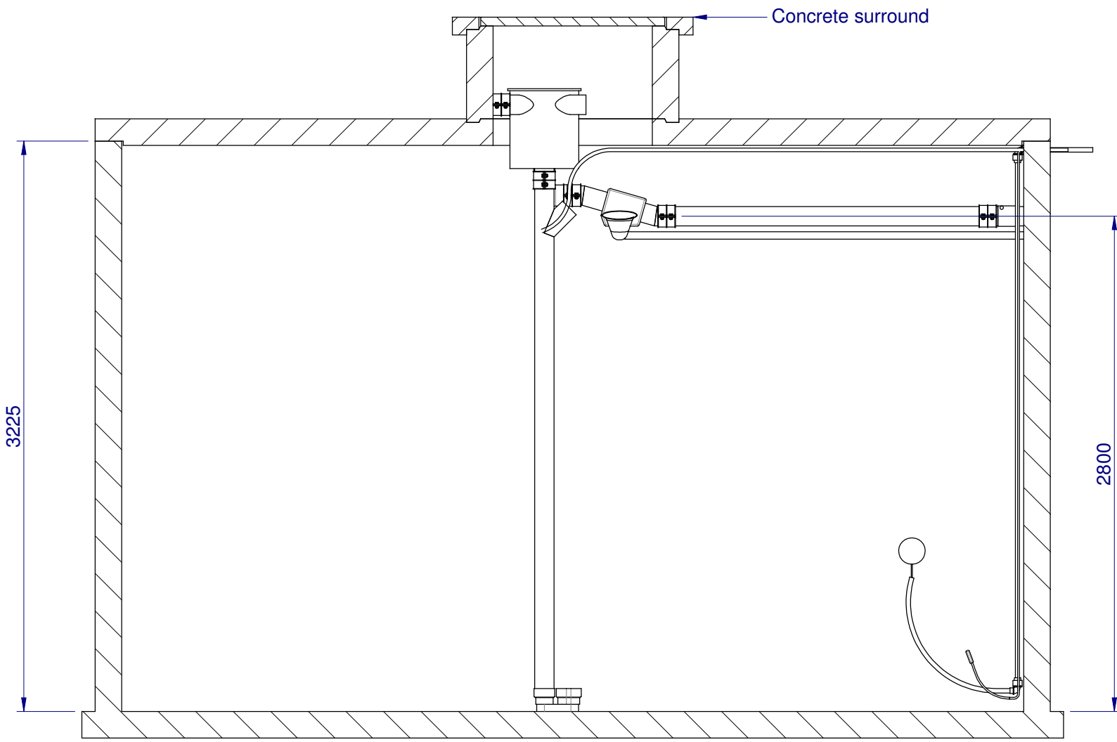
SECTION A-A
